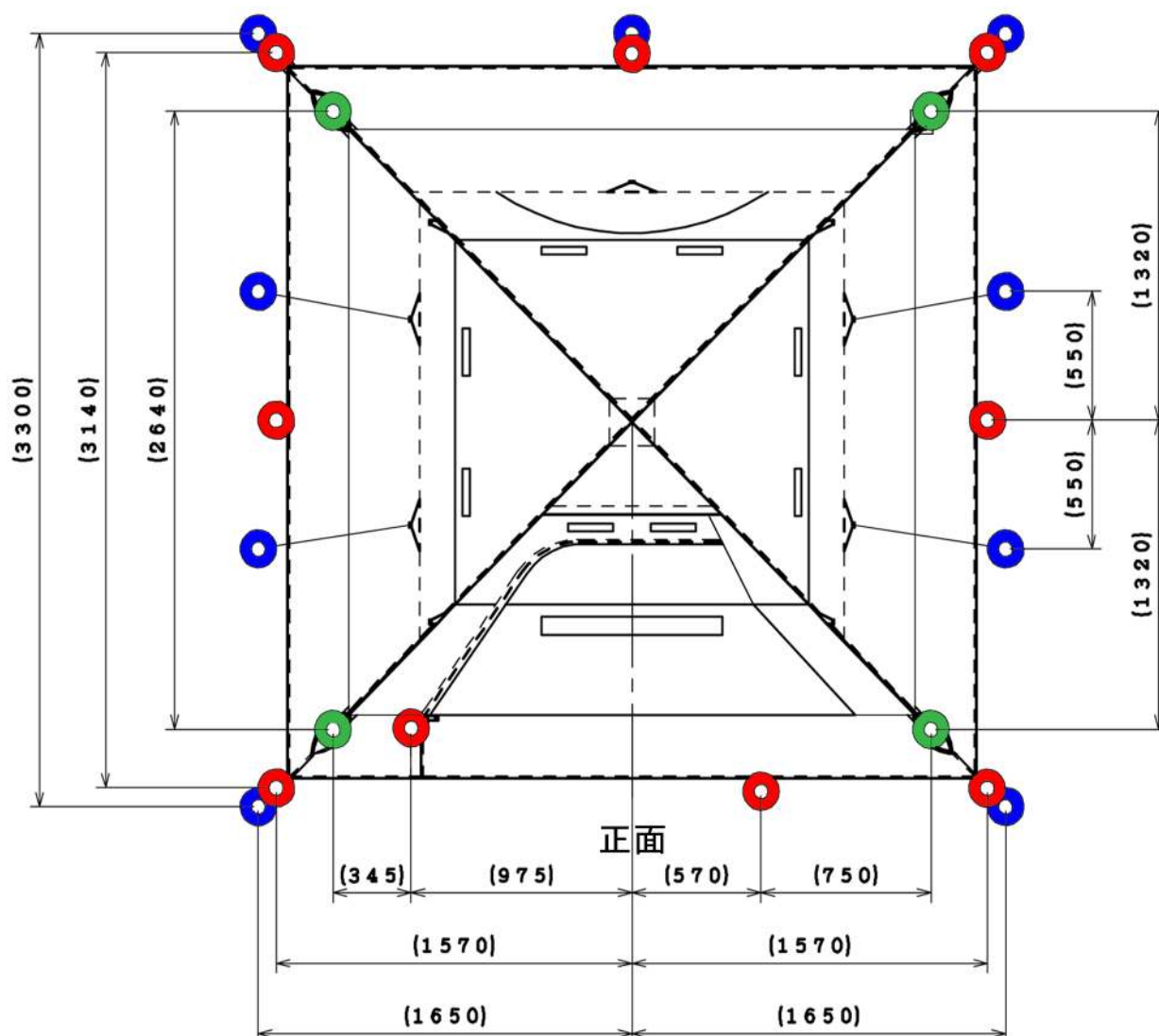
NT-TP260SET (災害用トイレ 大型テントセット)
