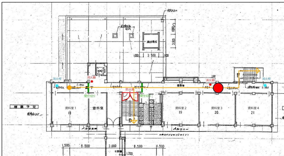
火災警報器設置位置図
