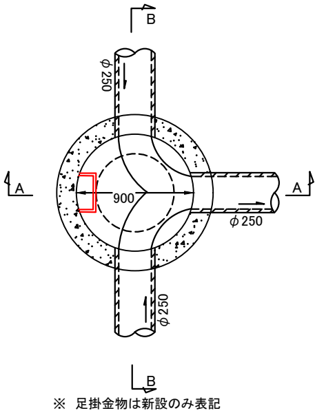
平面図
