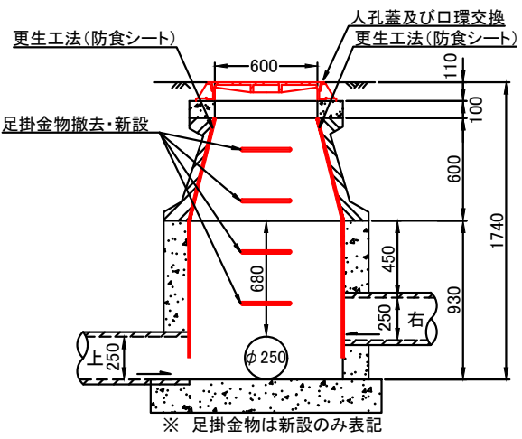
B - B 断面図
