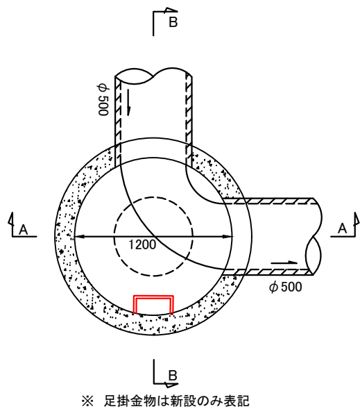
平面図
