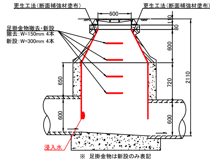
A - A 断面図
