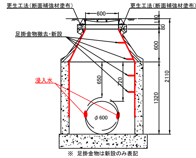
B - B 断面図
