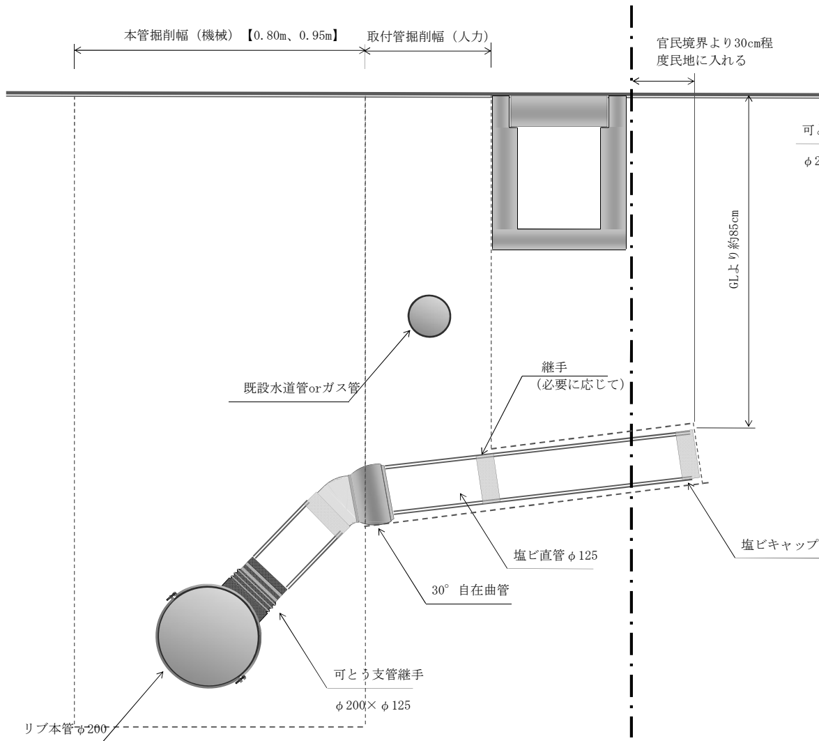
縦断面図
