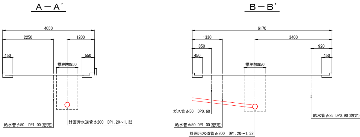
断面図 縮尺 1:50
