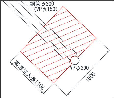
【薬注詳細図】
