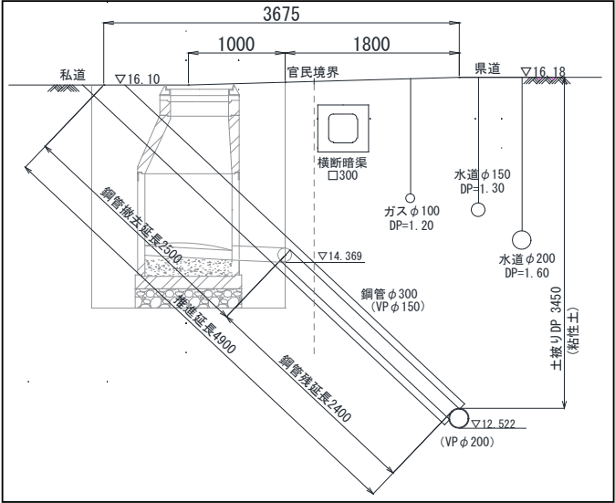
【参考推進断面図】
