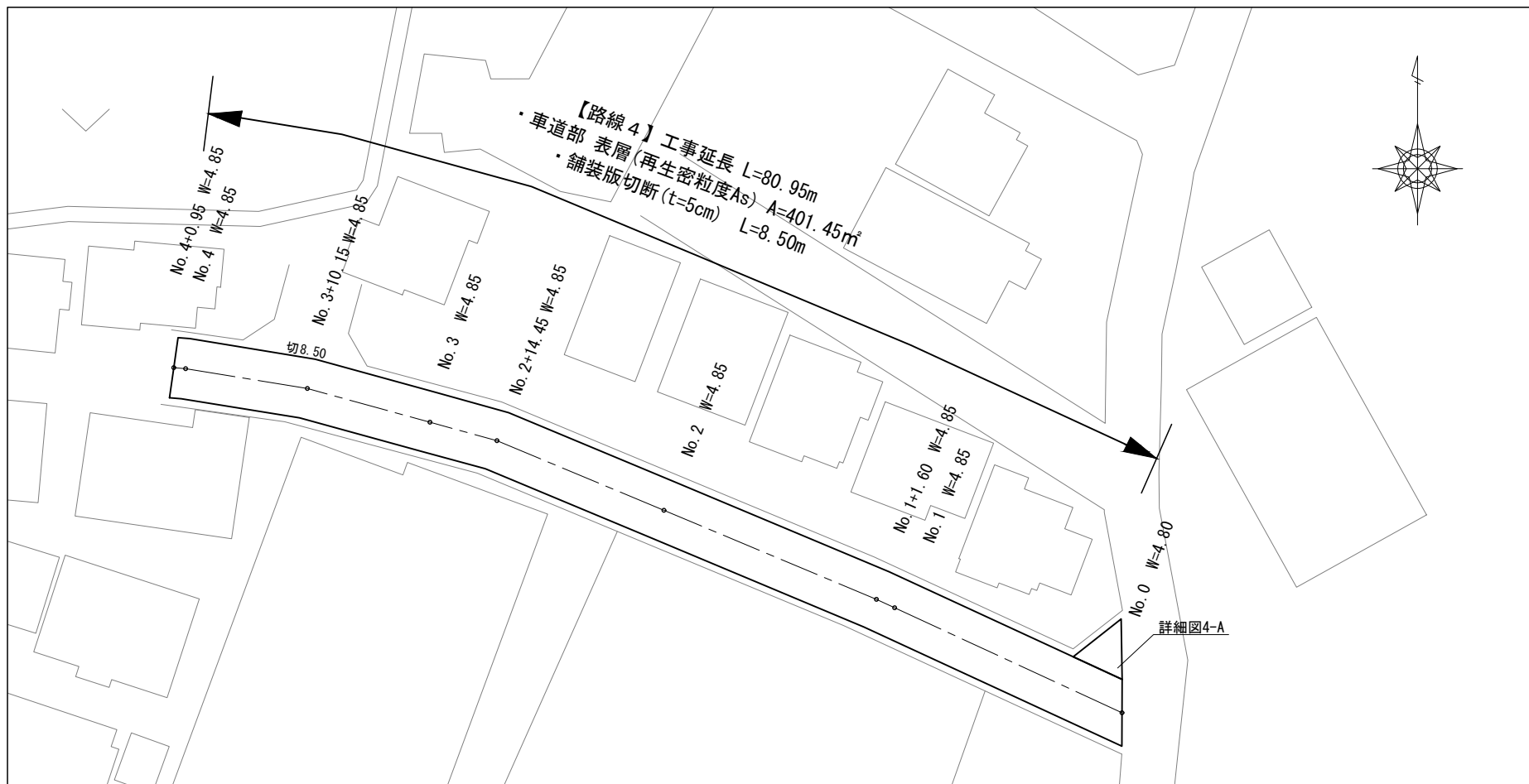
平面図 S=1:500 (路線 4)
