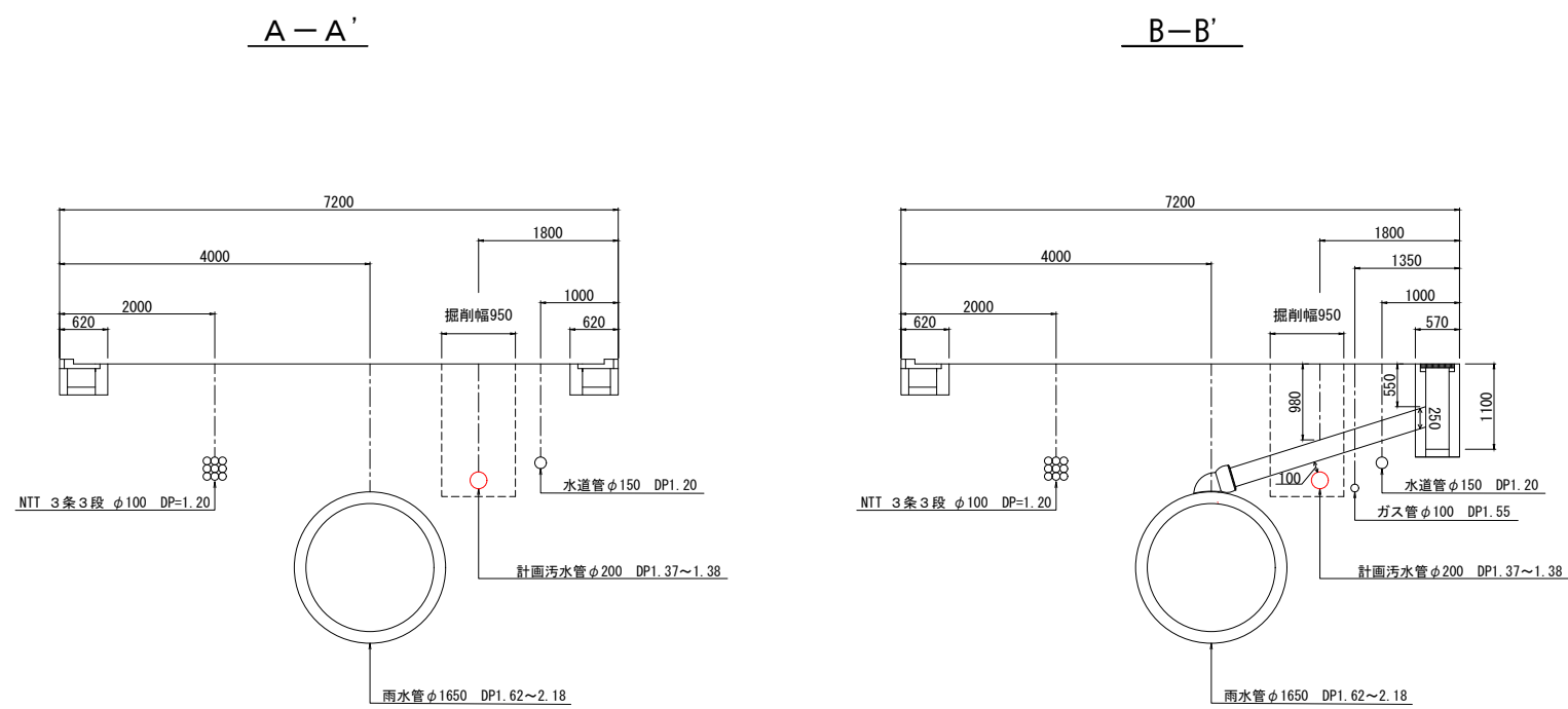
横断面図 縮尺 1:50
