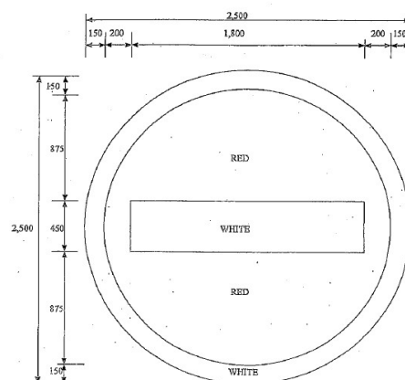
寸法図
