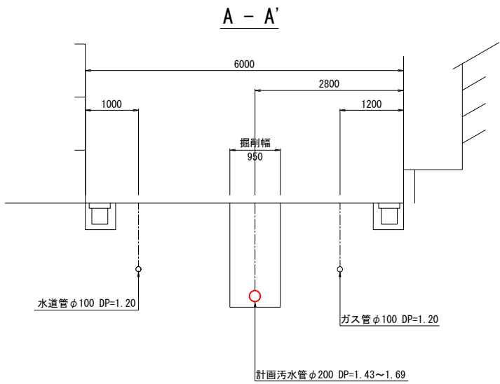
横断面図 縮尺 1:50
