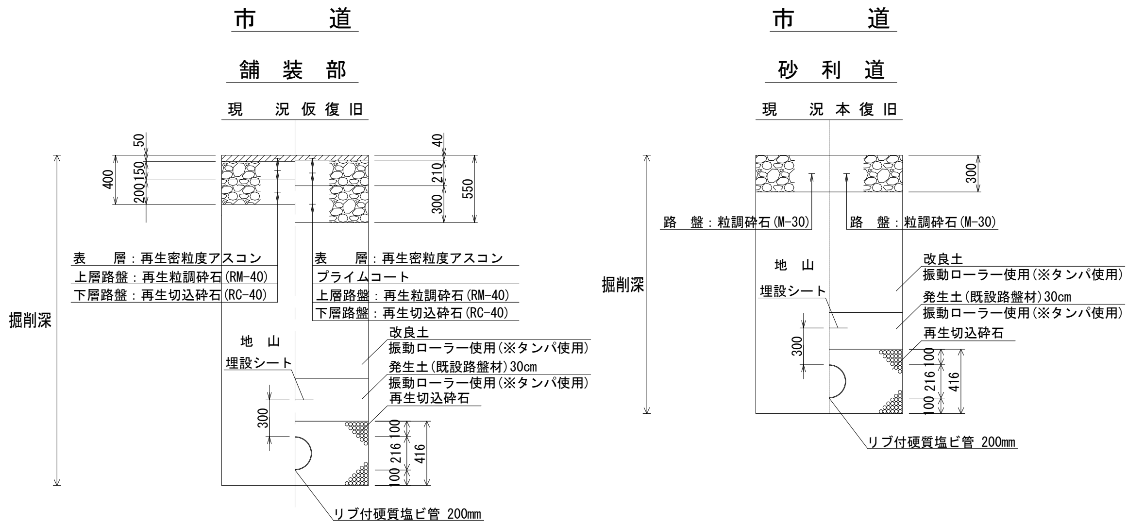
舗装構成図 縮尺 1:30
