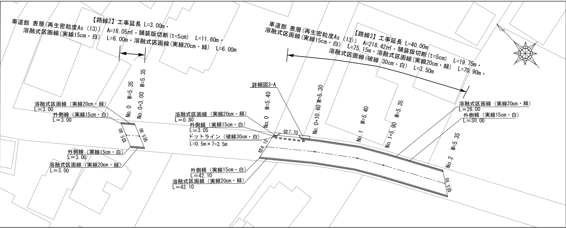
平面図 S=1:500
