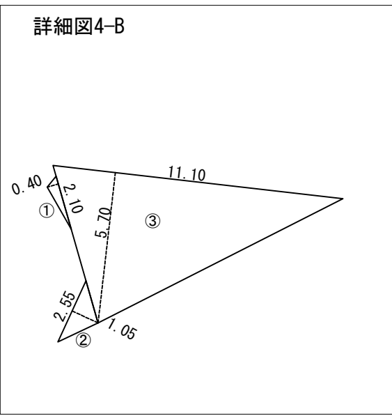
詳細図 S=1:200
