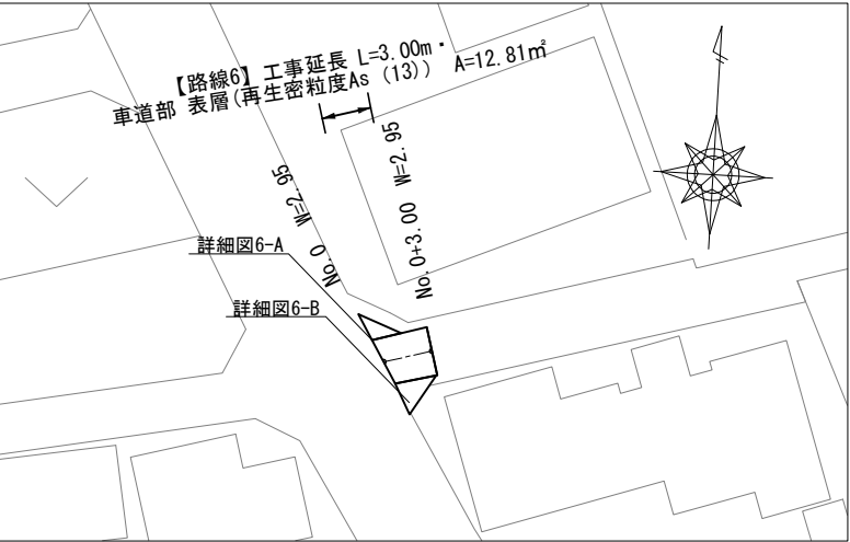
詳細図 S=1:100
