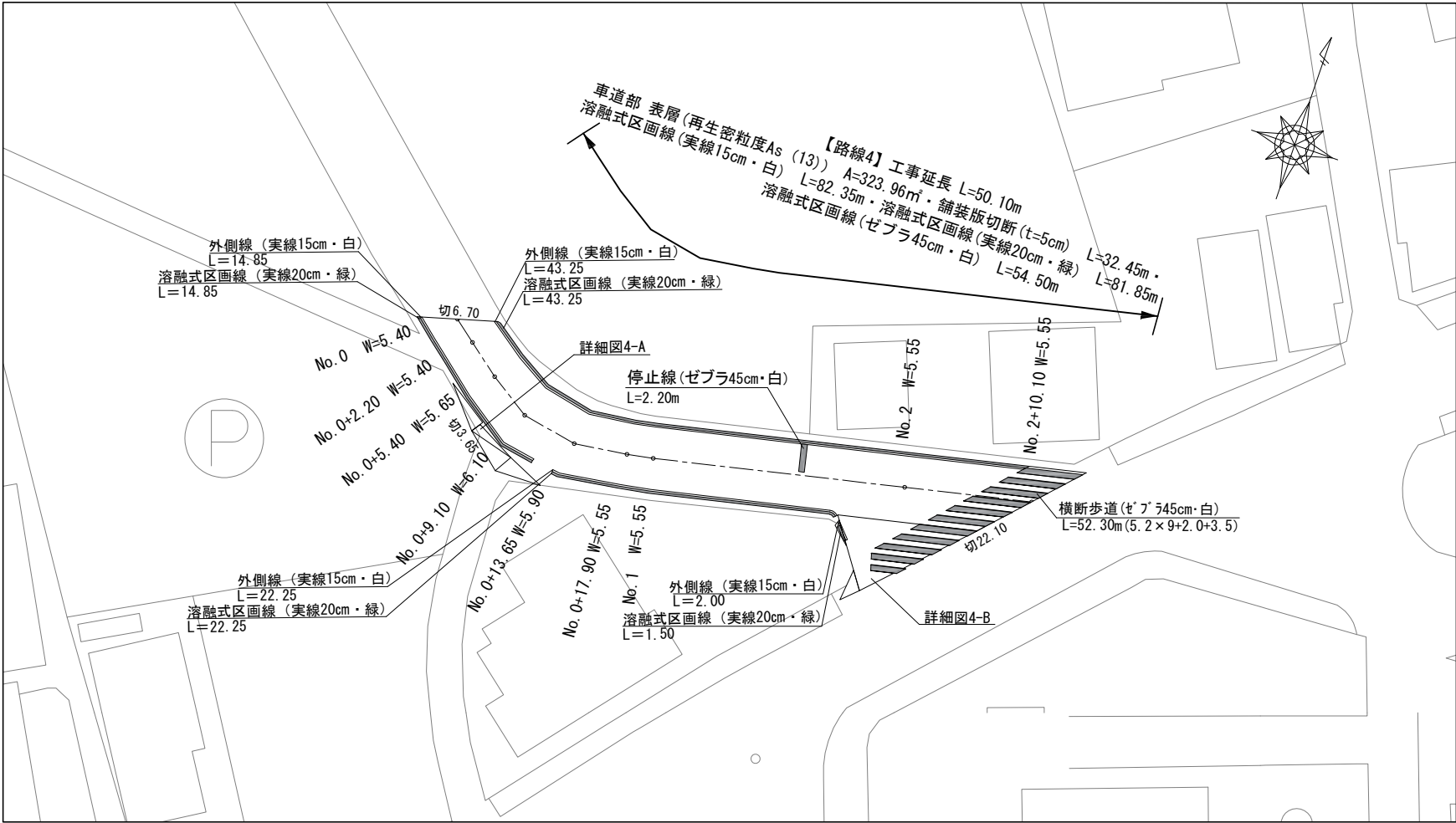
平面図 S=1:500
