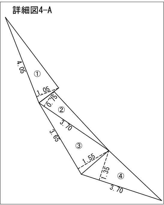
詳細図 S=1:200
