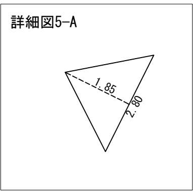
詳細図 S=1:100
