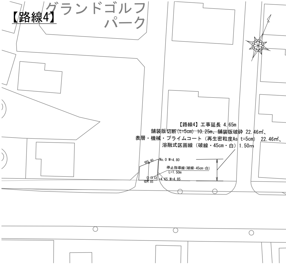
平面図 S=1:500
