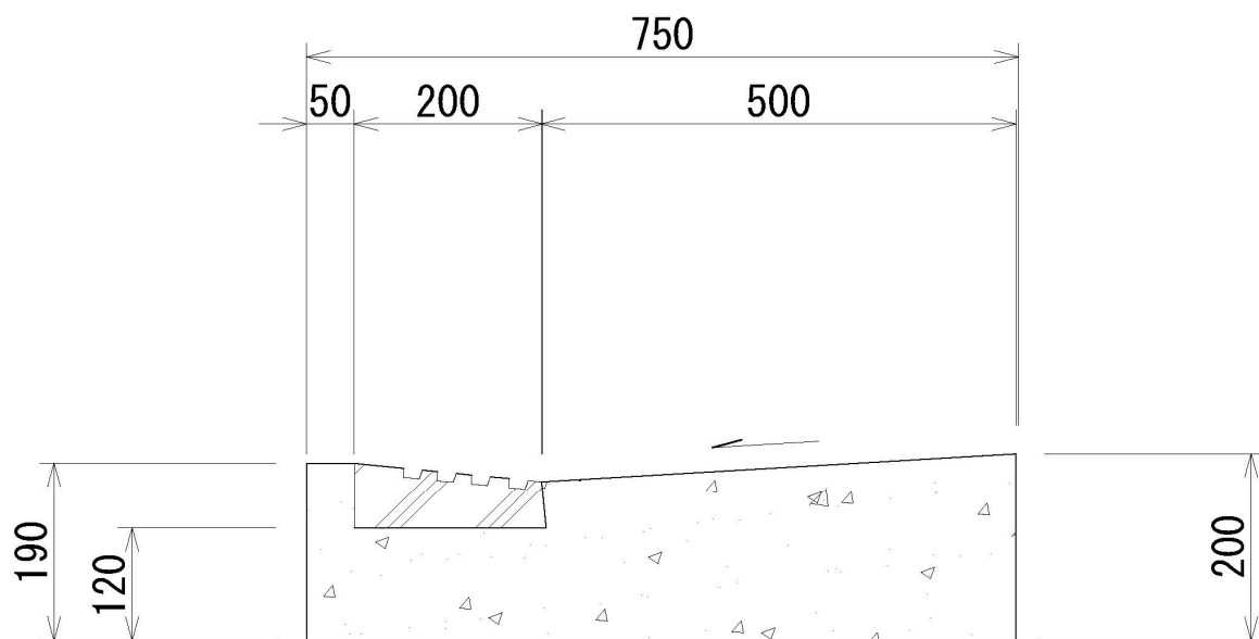
既設上層路盤
