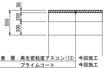
組成図 S=1:50
