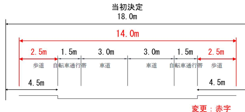
【道路標準断面図】 幅員変更区間 (県道さいたま菖蒲線から伊奈町整備済道路までの区間)
