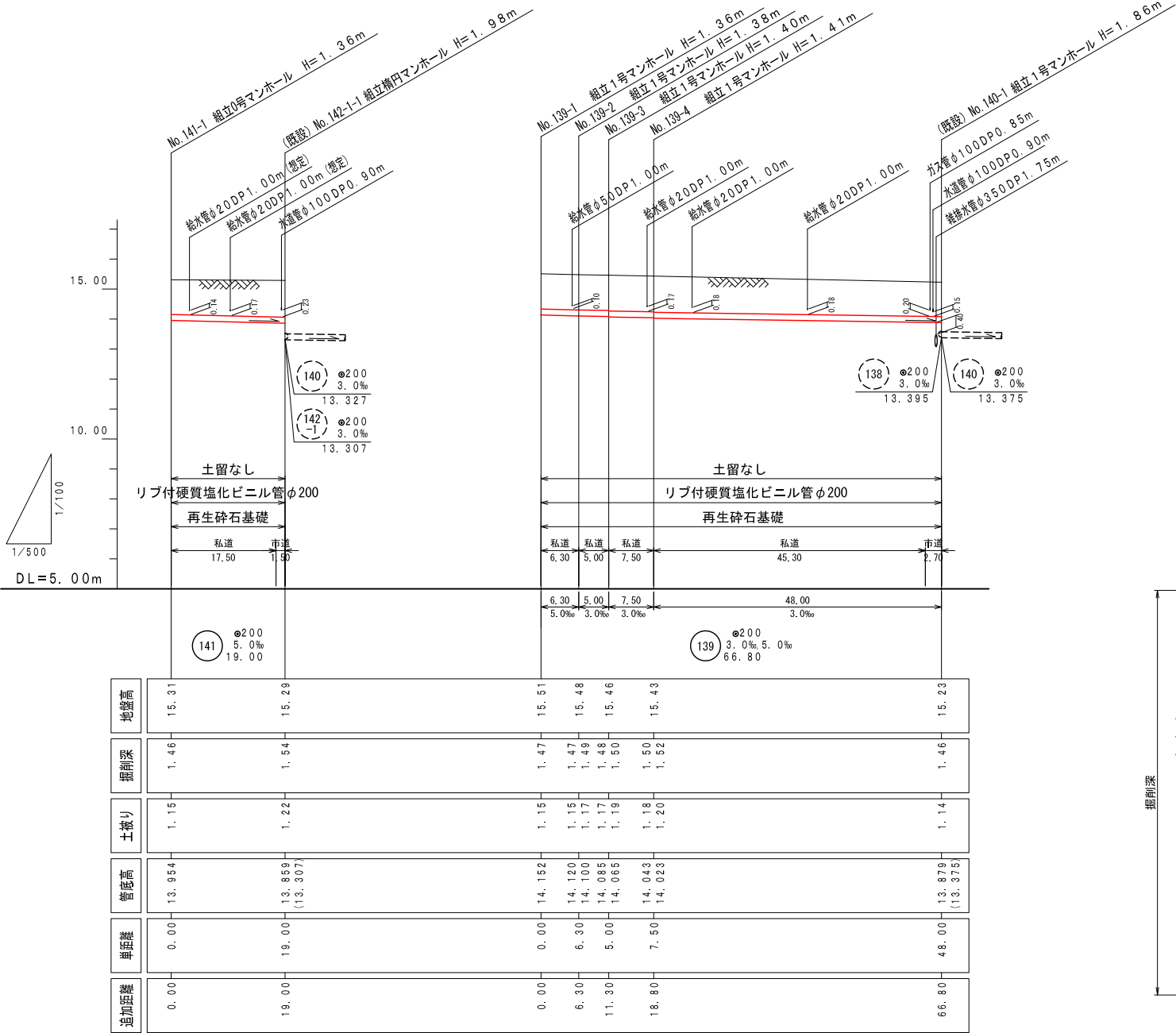
縦断面図 縮尺 縦 1:100 横 1:500
