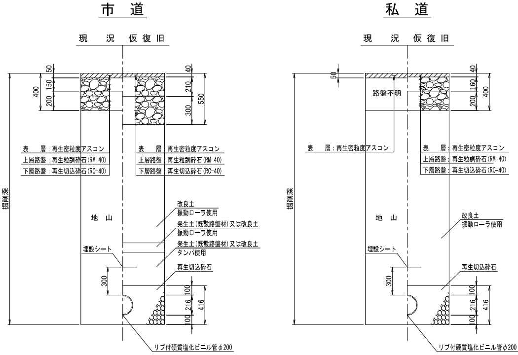
舗装組成図 縮尺 1:20
