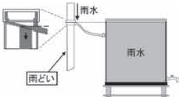
タンクの構造。雨どいとタンクをホースでつなげてタンクに雨を貯めます。
