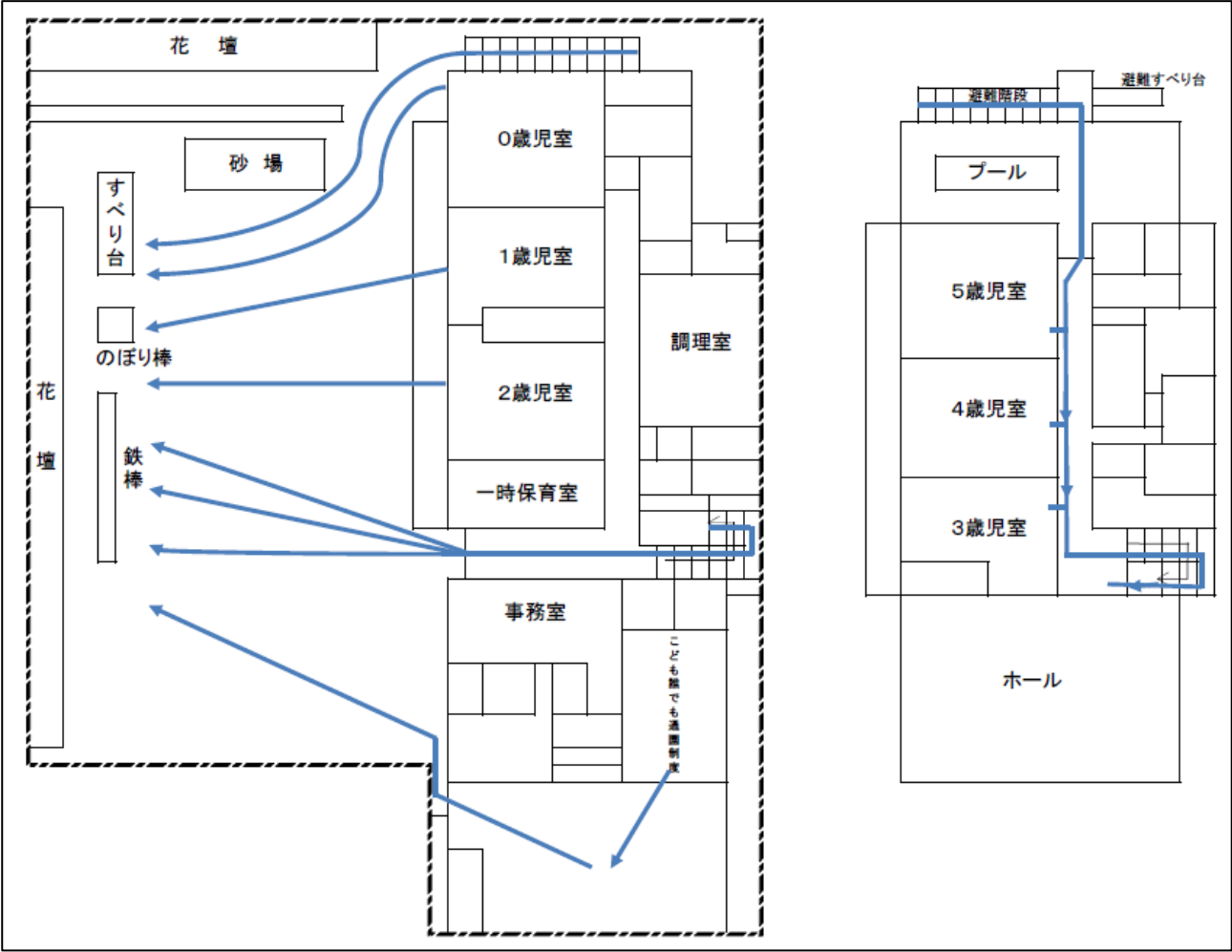
避難経路図
