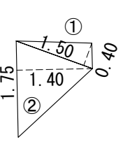
打換3-D
