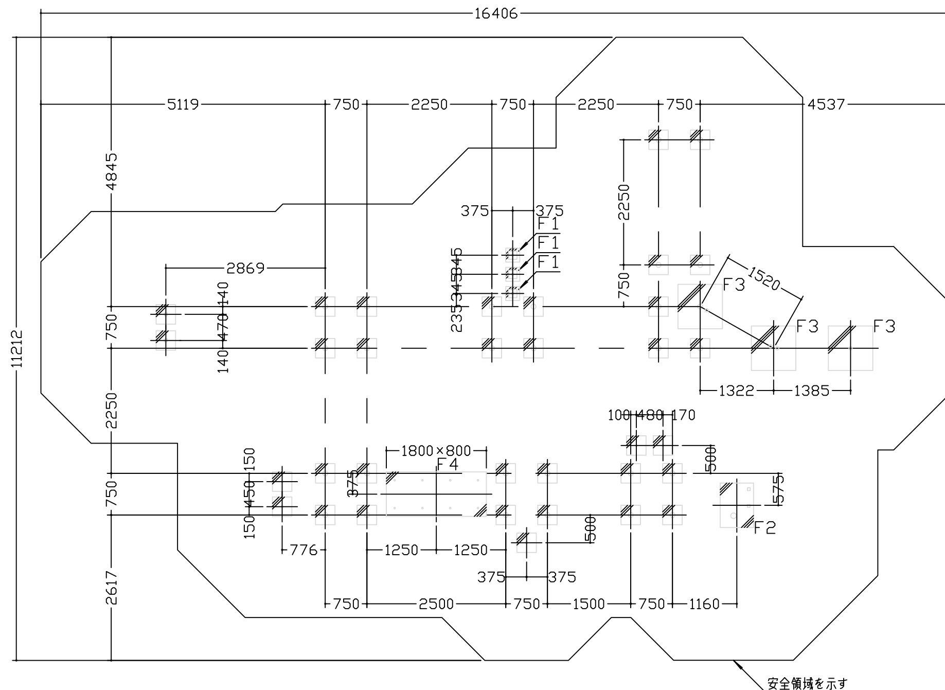
基礎伏図 S=1/70
