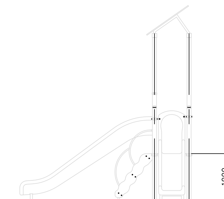
B 視立面図 S=1/50
