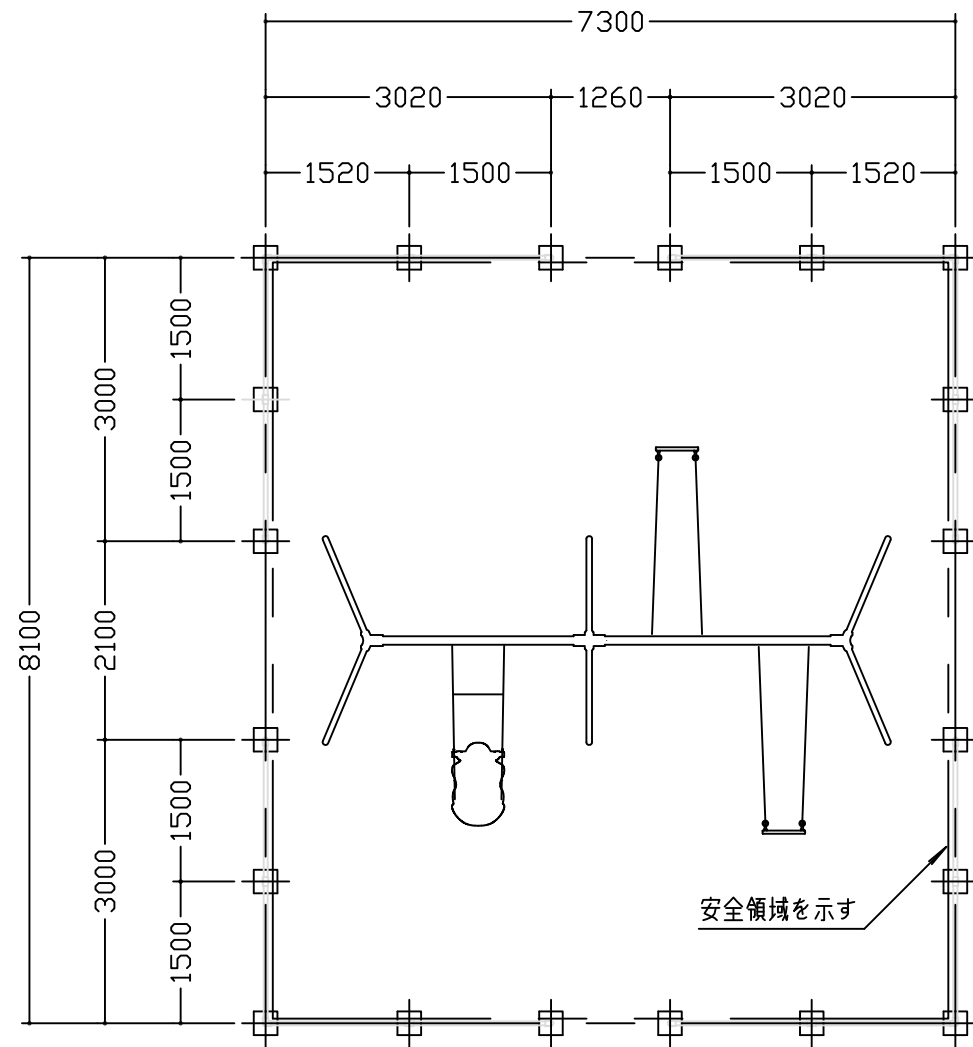
平面図 S = 1 / 80
