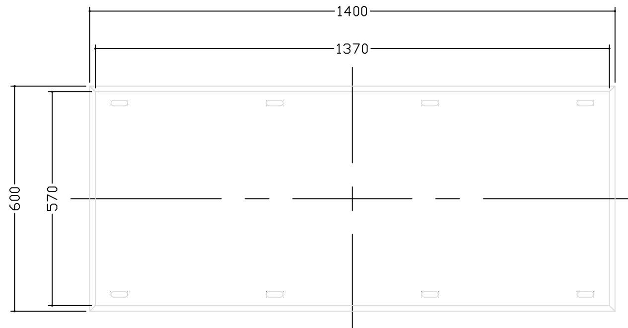
平面図 S = 1 / 1 0
