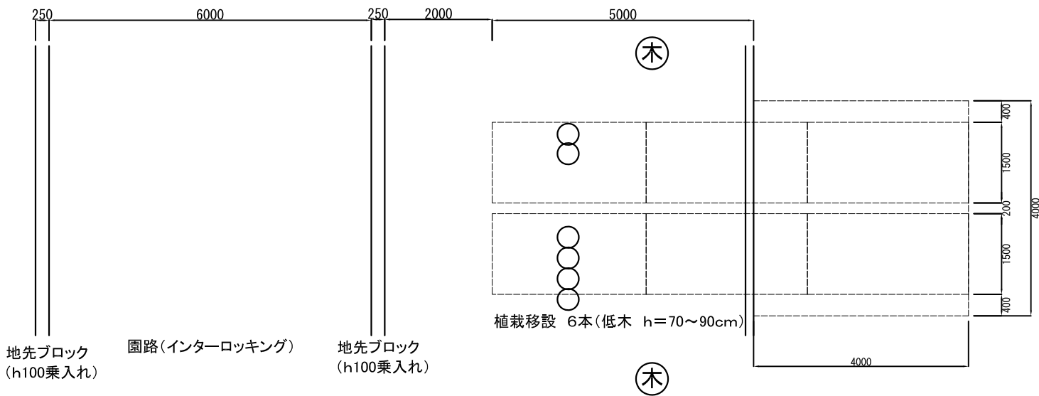
既設平面図 1/100
