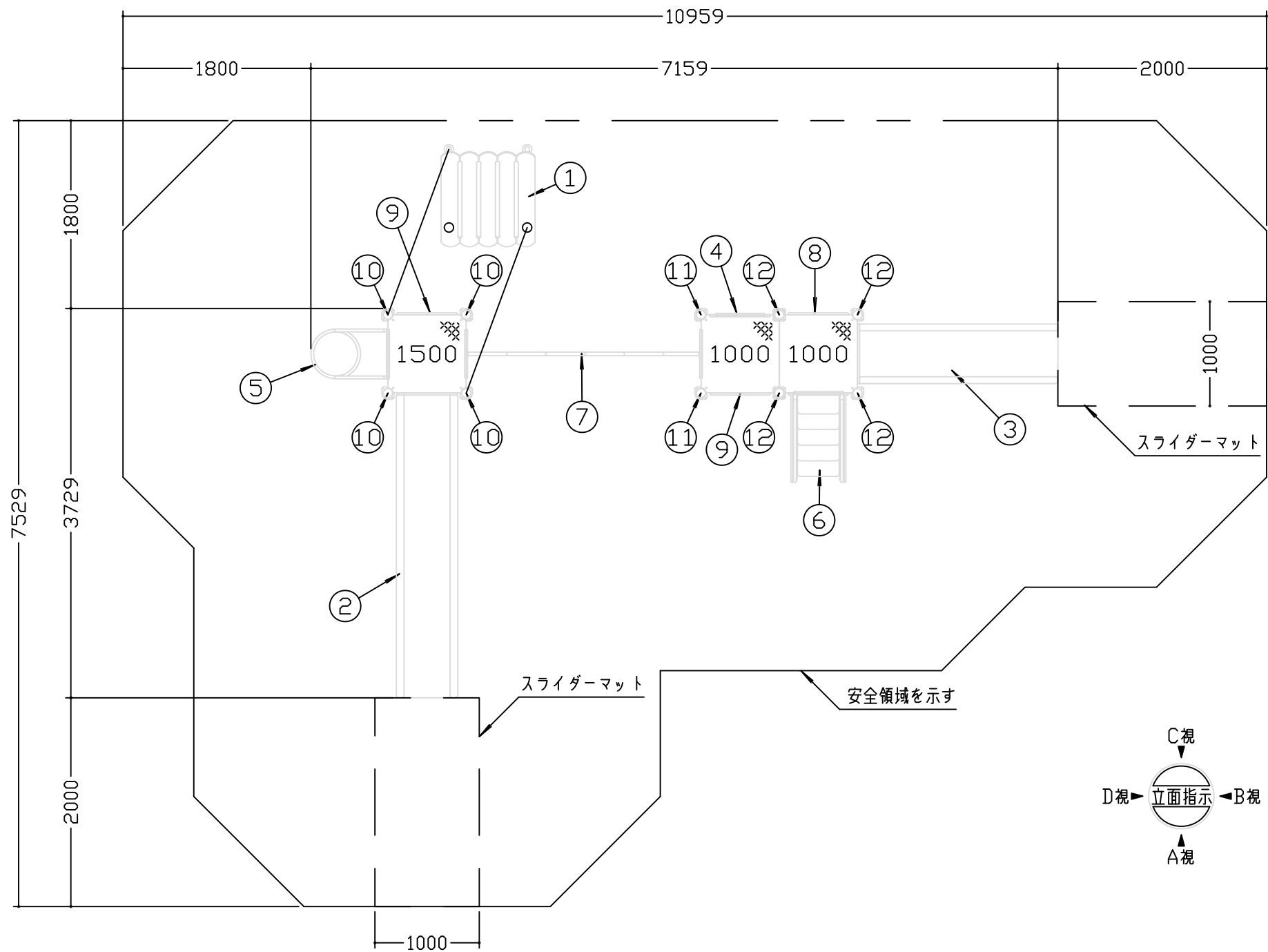
平面図 S=1/50
