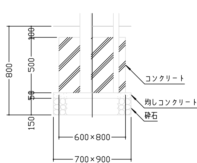
F2基礎断面詳細図 S=1/20
