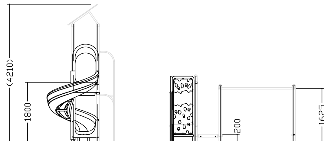
B 視立面図 S=1/70
