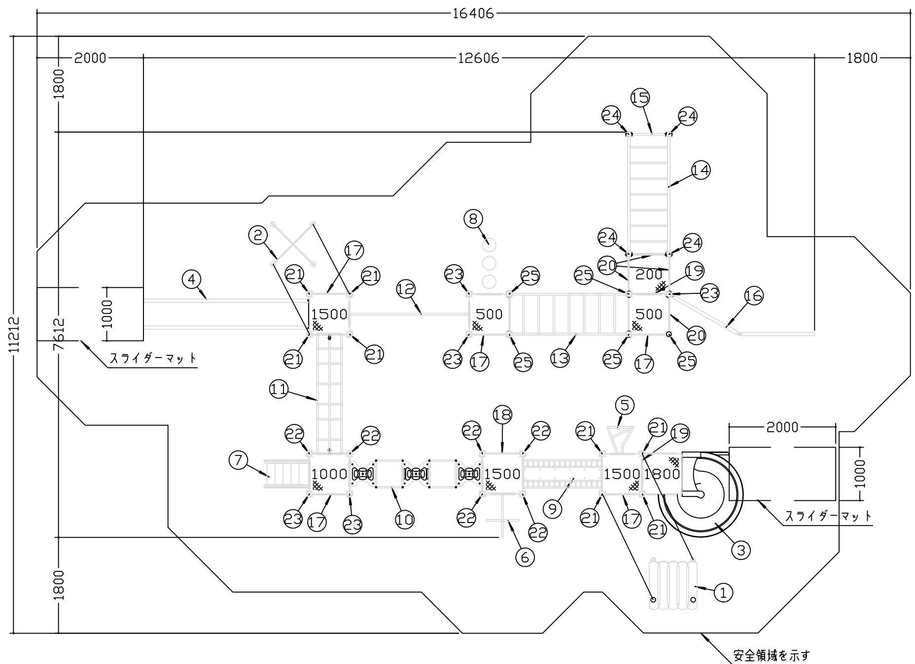
平面図 S=1/70
