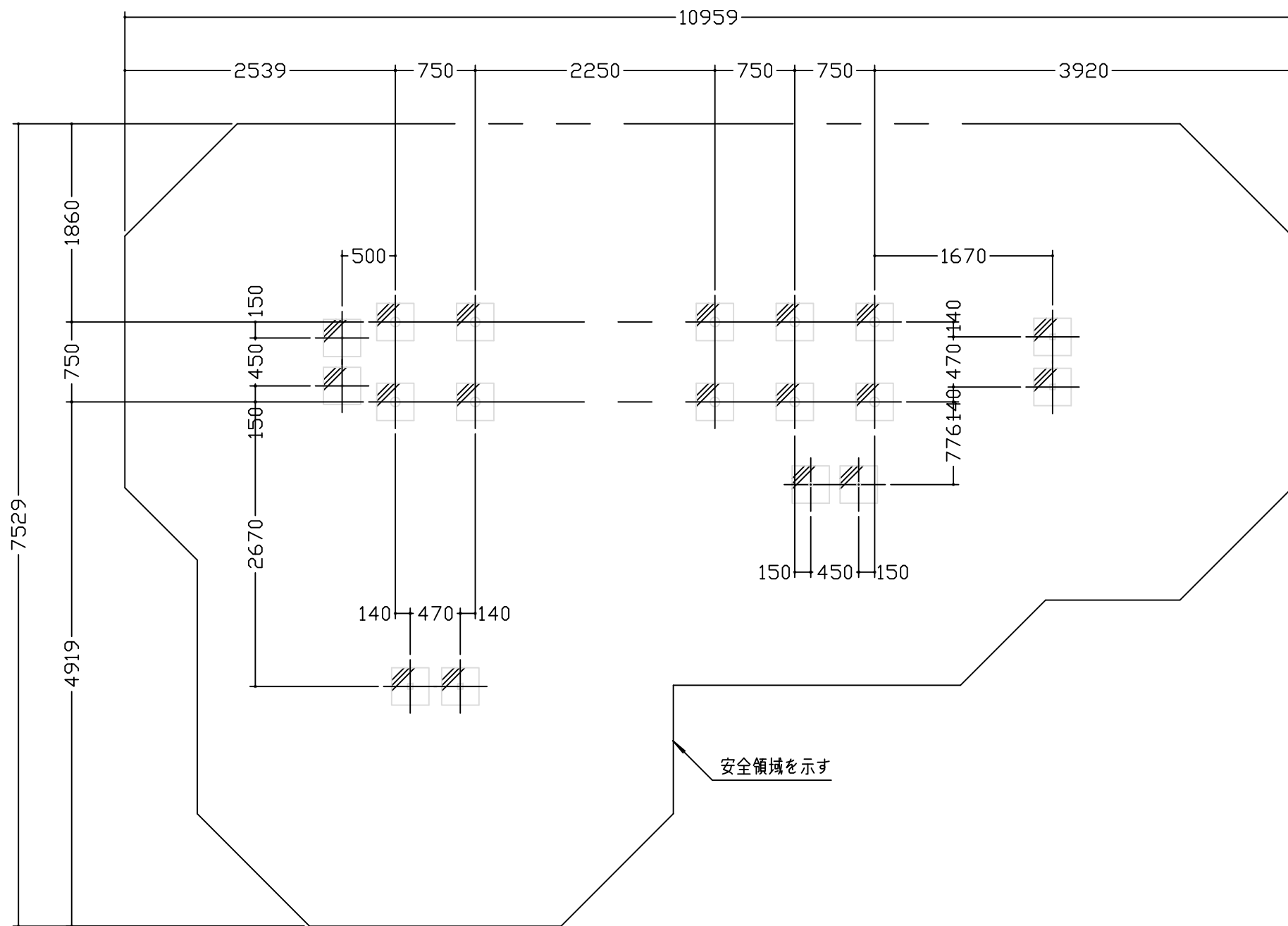
基礎伏図 S=1/50
