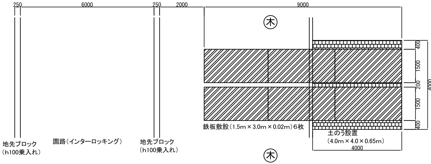
工事用道路位置図 1/2000
