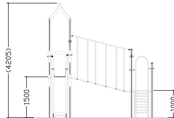
D 視立面図 S=1/70
