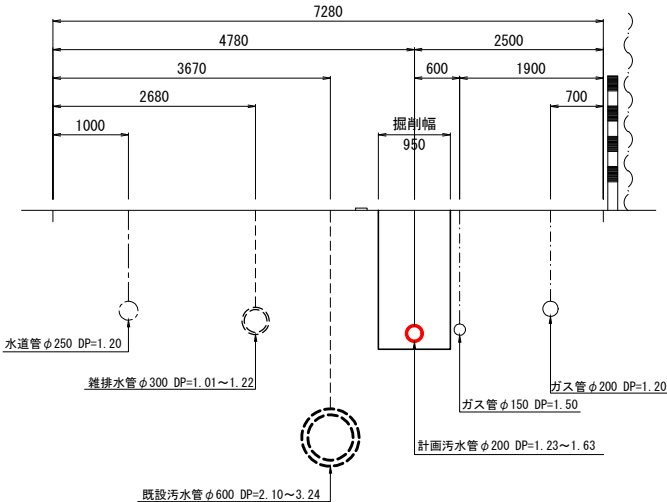
E-E' No. 1-1-3人孔部
