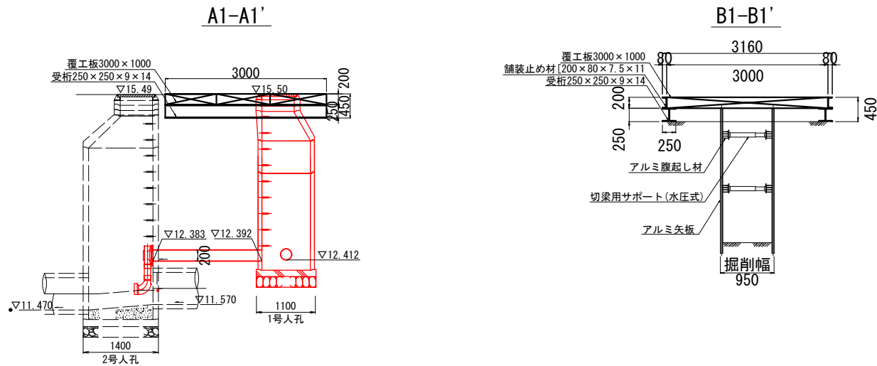
No. 3-1-3人孔部
