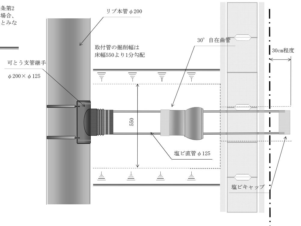
断面図
