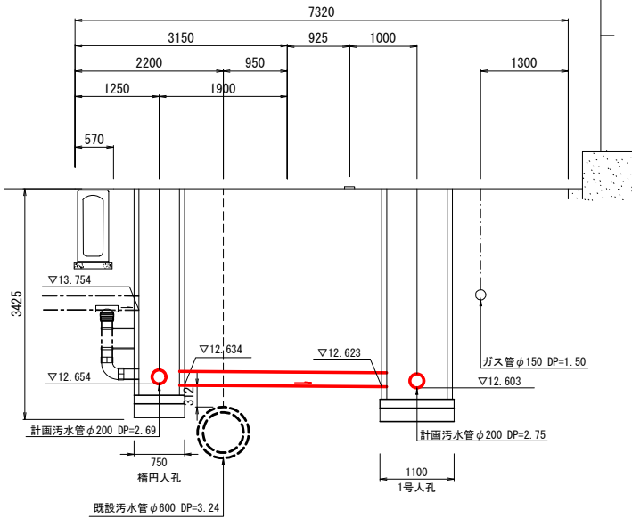
H-H' No. 3-1-1人孔部
