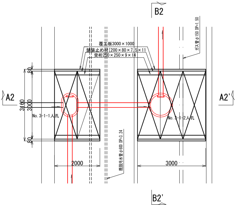
No. 3-1-1人孔部
