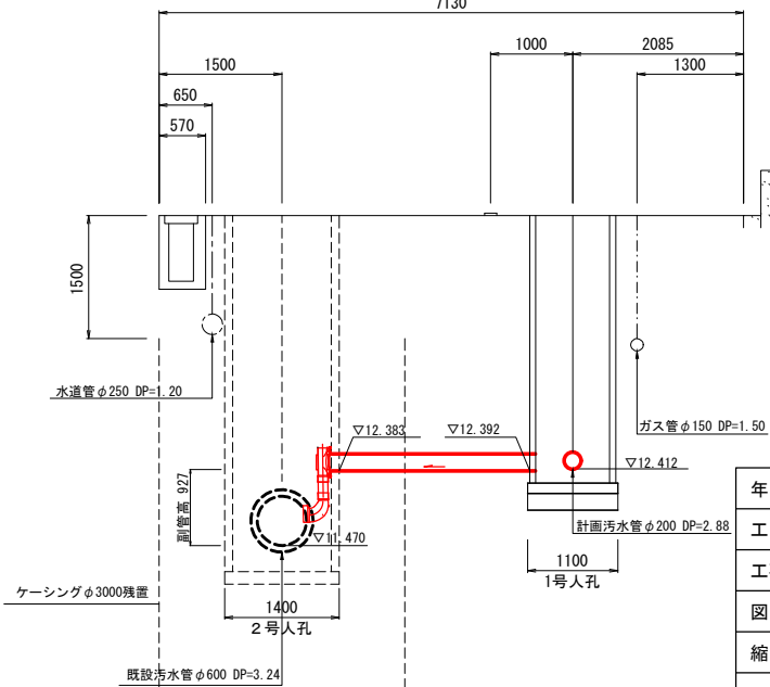
I-I' No. 3-1-3人孔部
