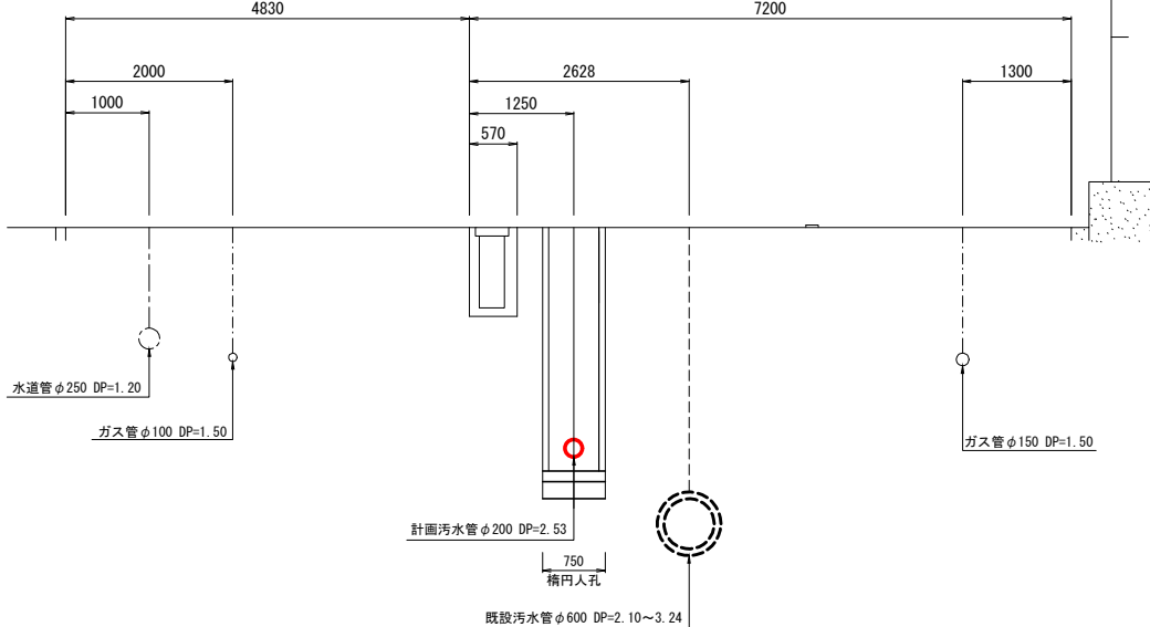
I-I' No. 3-1-3人孔部
