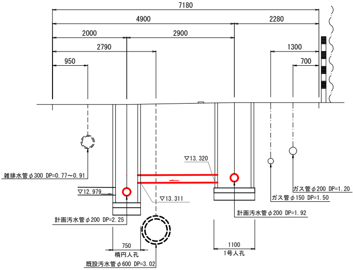
H-H' No. 3-1-1人孔部
