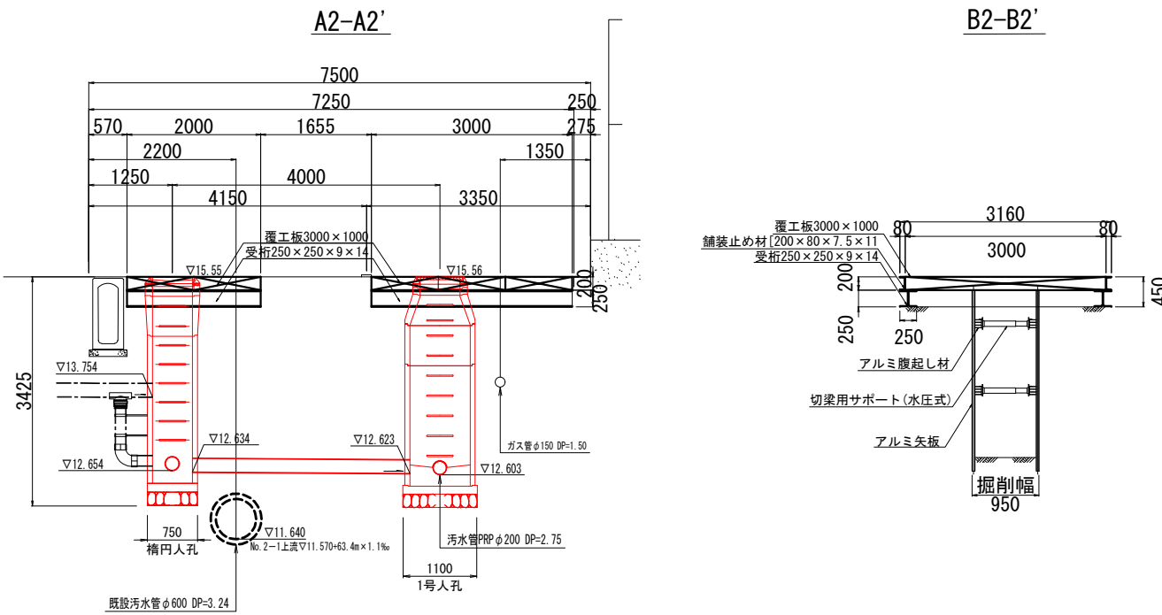
No. 3-1-1人孔部
