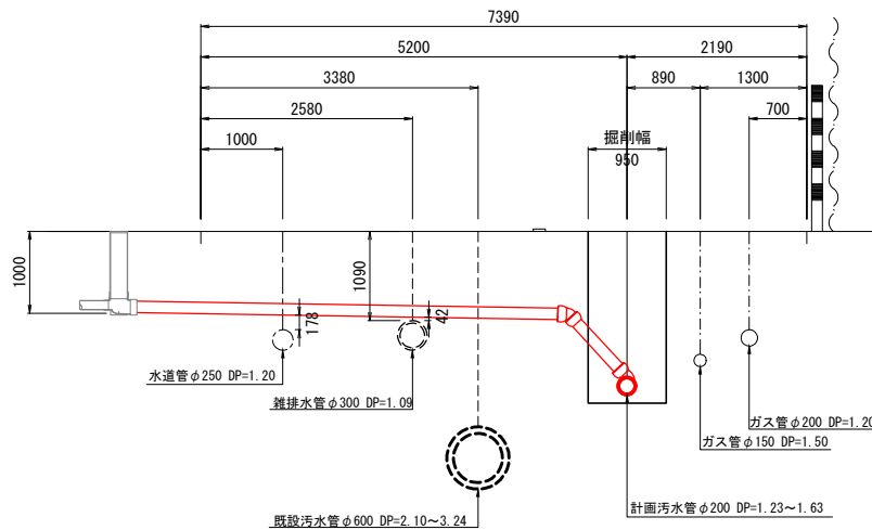
F-F' No. 2-1-2人孔部
