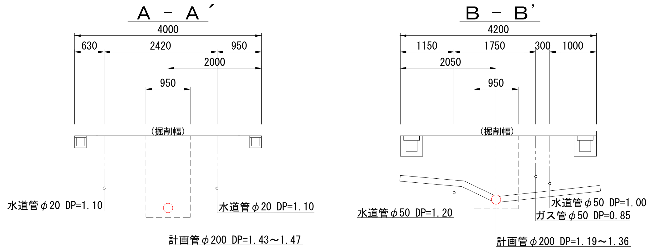
断面図 縮尺 1 : 50
