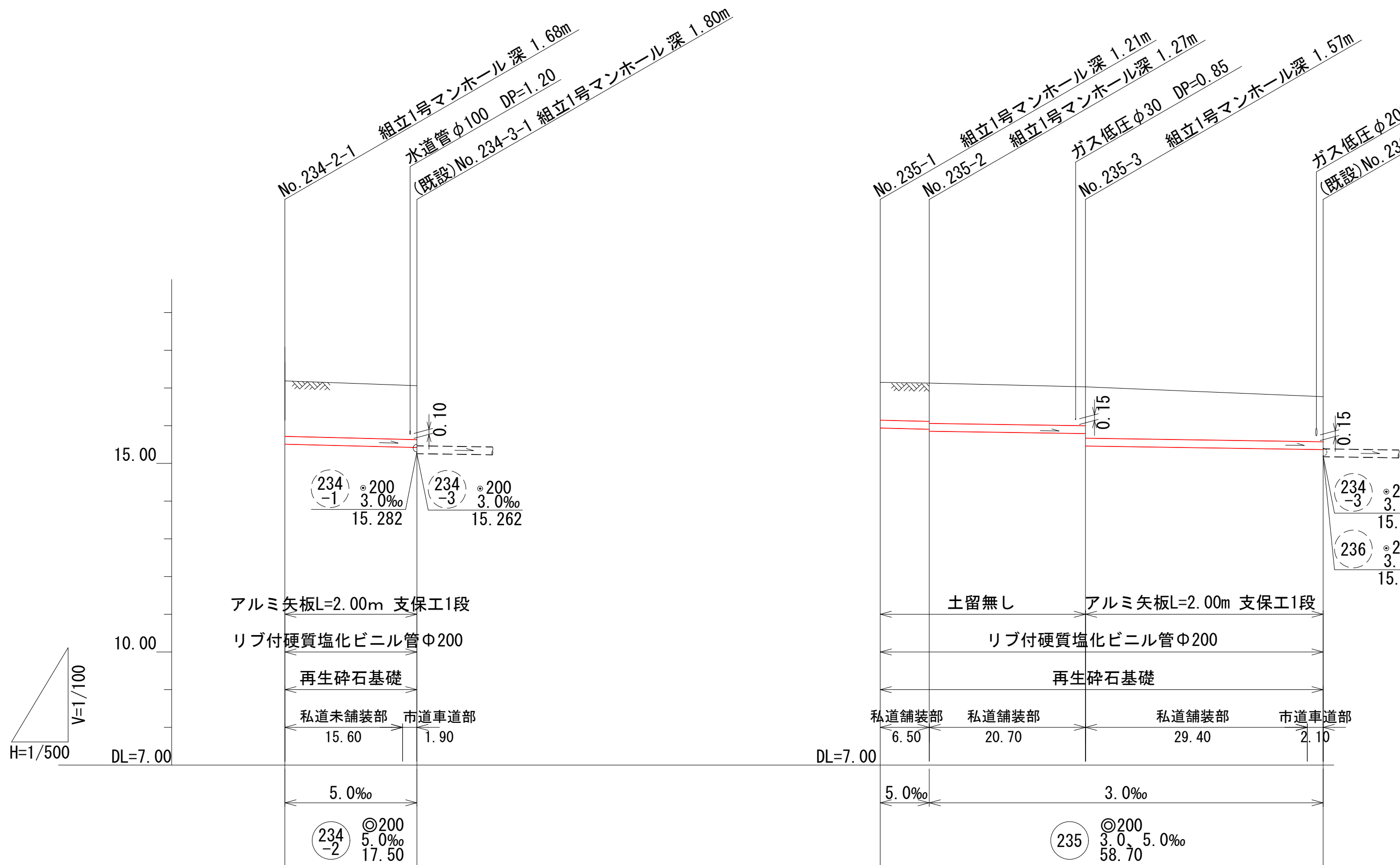
縦断面図 縮尺 縦 1 : 100 横 1 : 500
