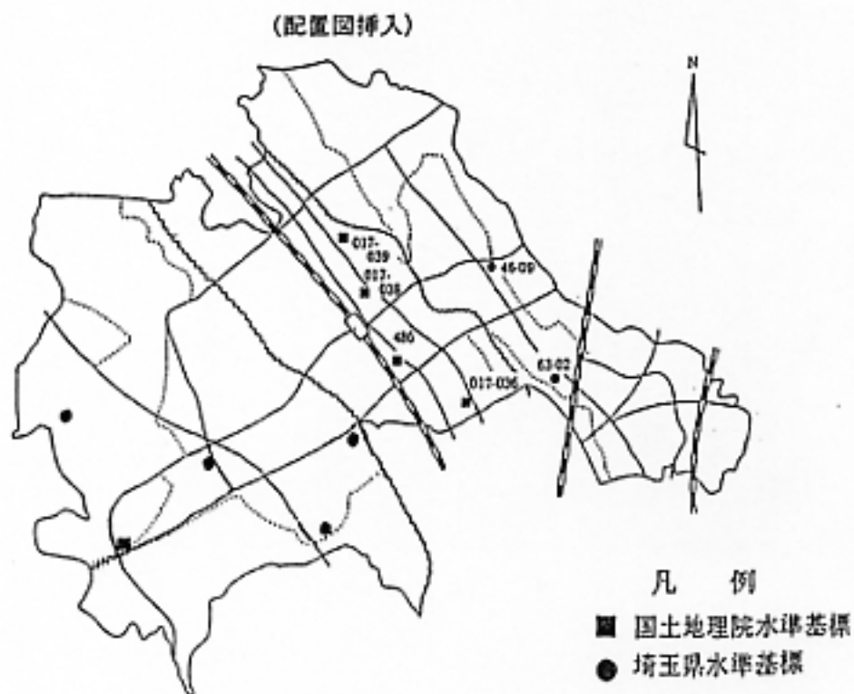
水準基標配置図
