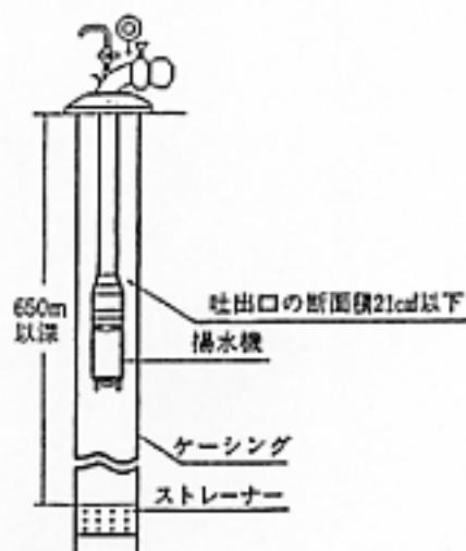
揚水施設の構造図 (許可基準)
